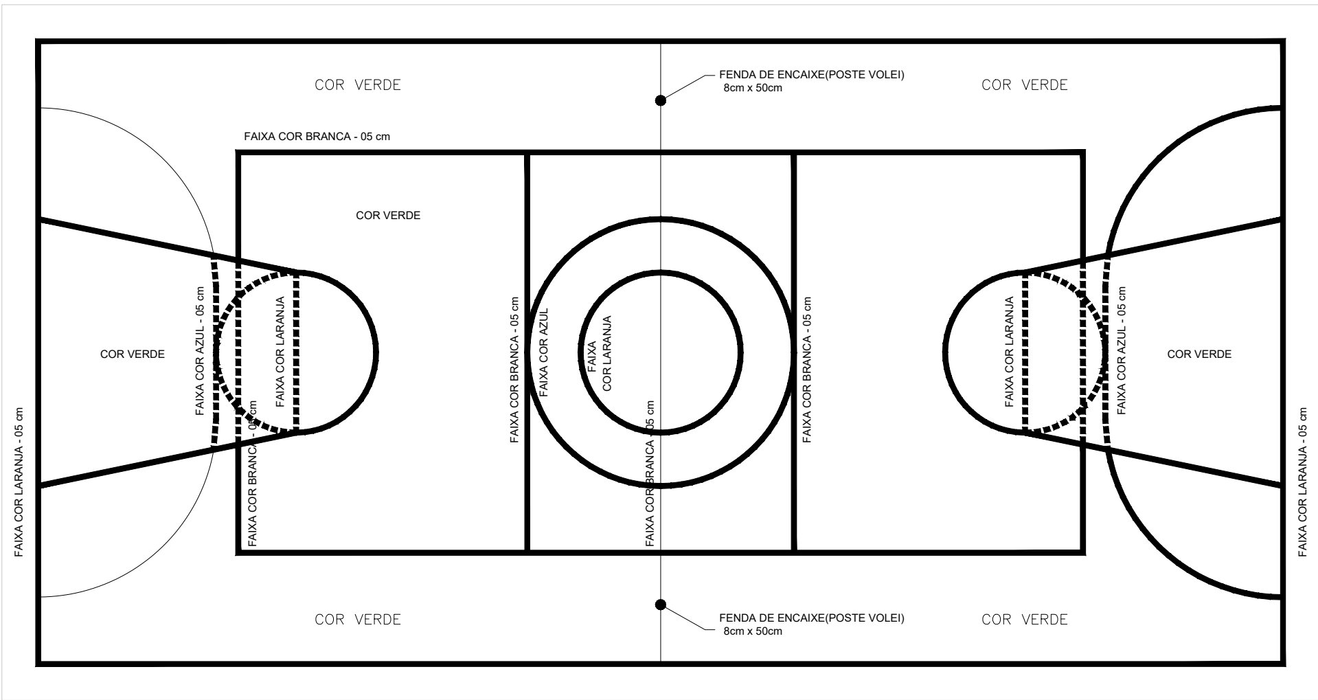
PINTURA DO PISO DA QUADRA - ÁREA INTERNA: 340,36M² ESC.: 1:100
