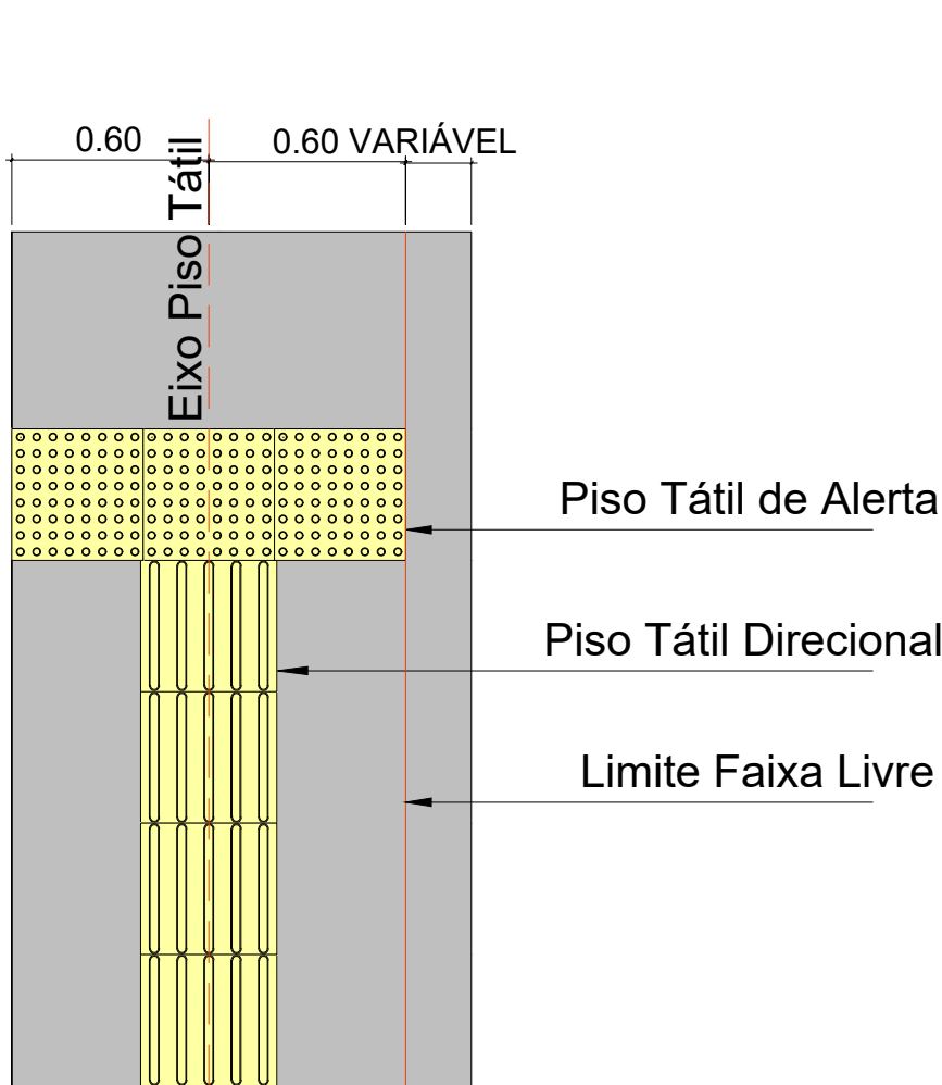
Detalhe 01 ESC.: 1:25
