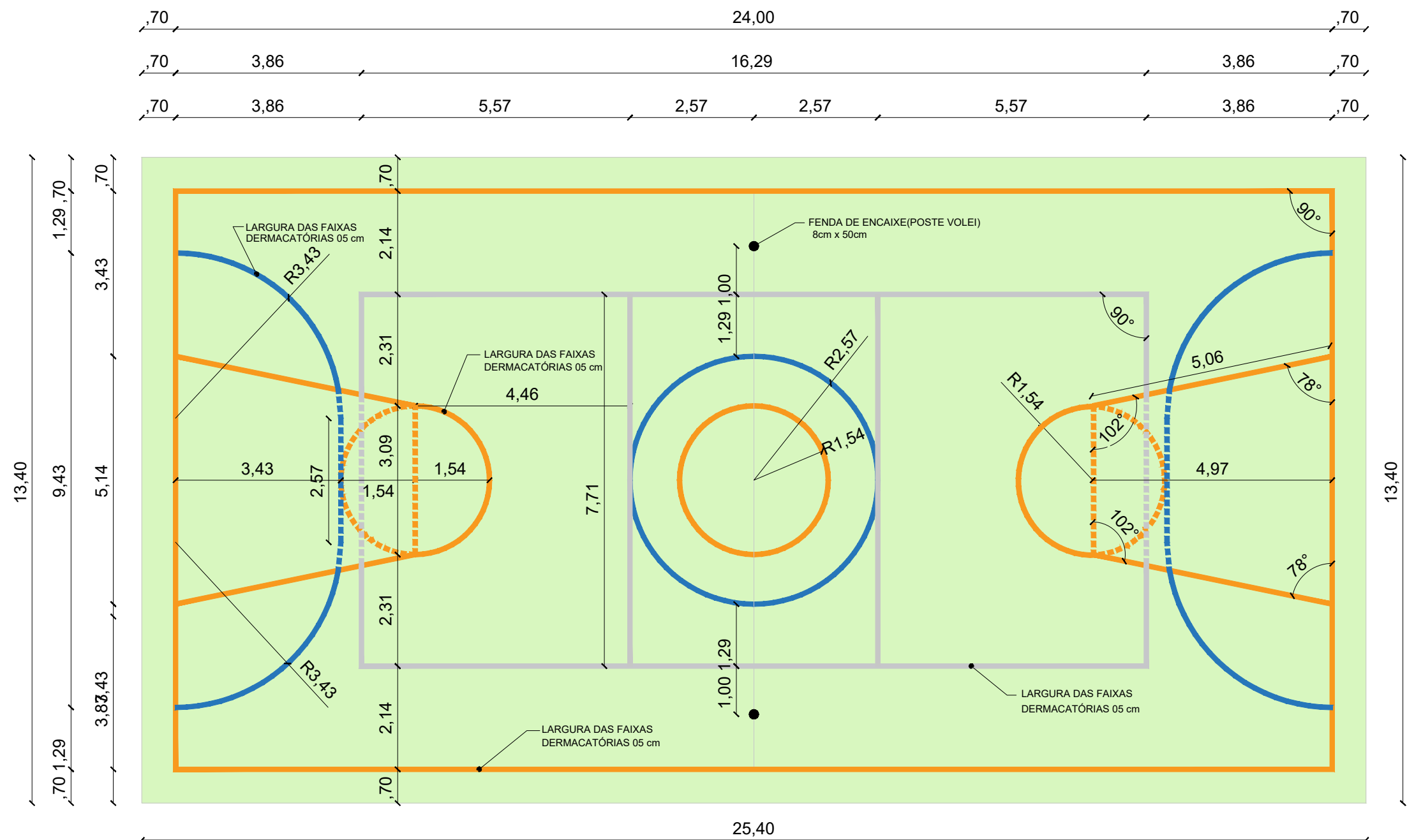
PINTURA DO PISO DA QUADRA - FAIXAS ESC.: 1:100
