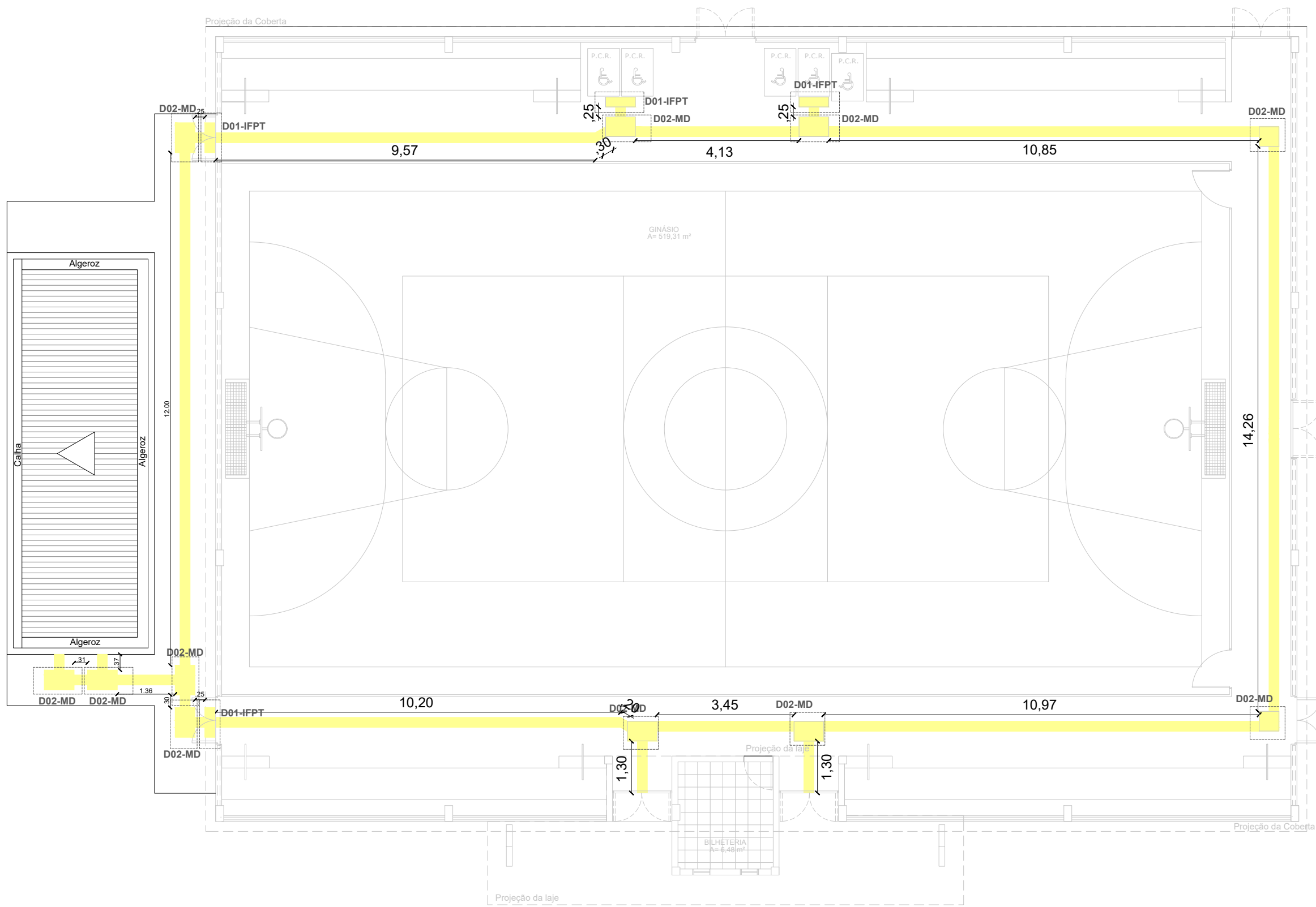
Planta Baixa - Acessibilidade escala 1/100
