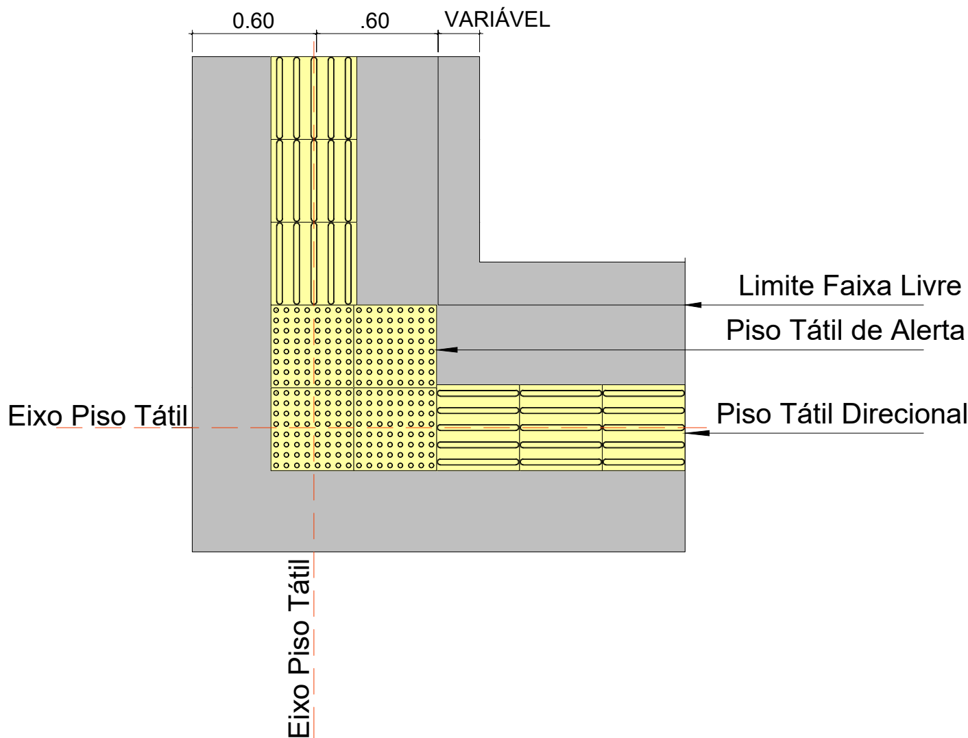
Detalhe 02 ESC.: 1:25
