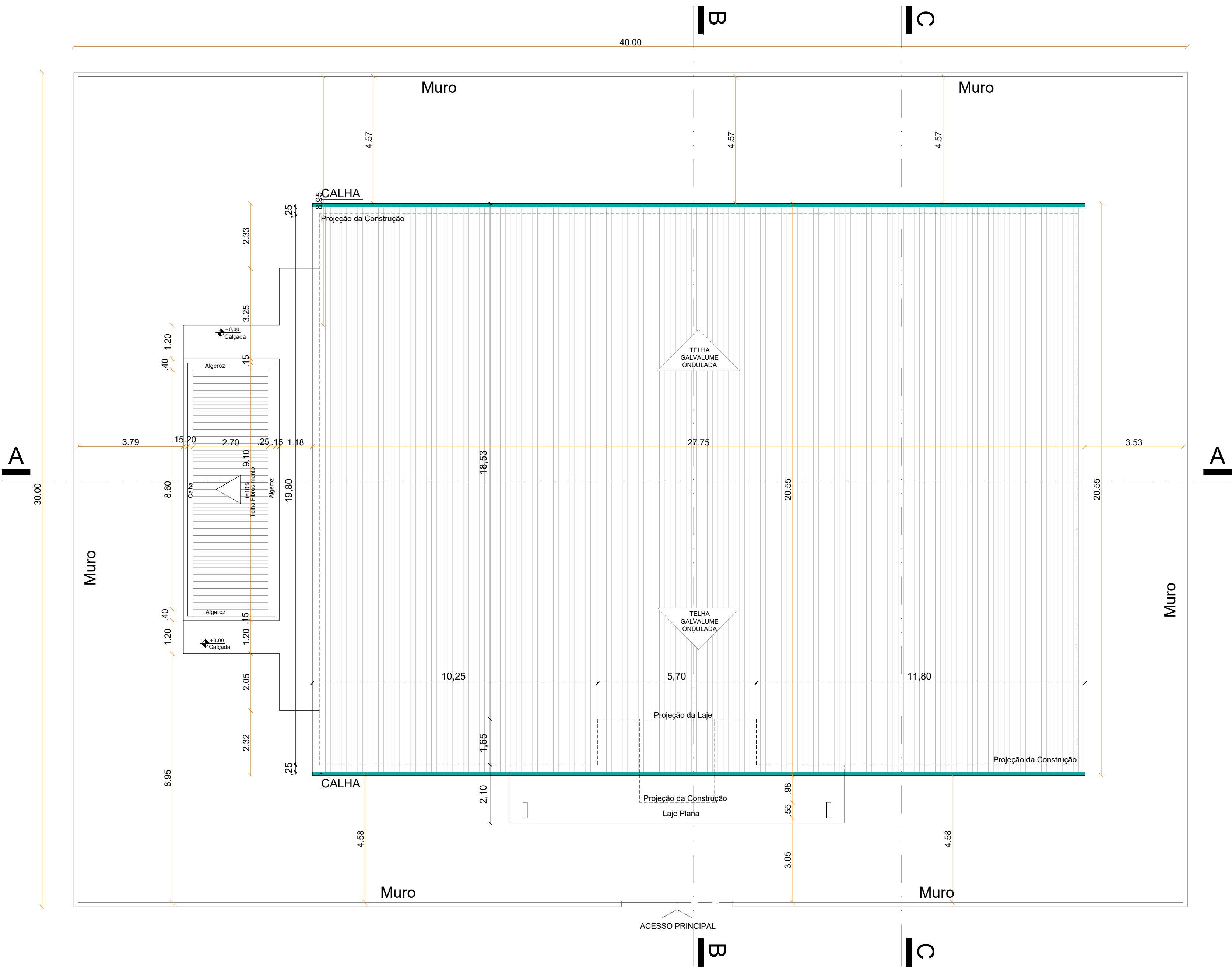
PLANTA DE COBERTA ESC.: 1:100
