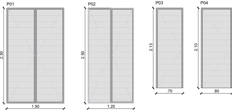
DETALHE 01 - ESQUADRIAS ESC.: 1:50
