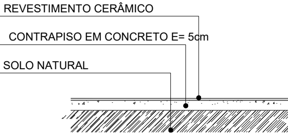
DETALHE 02 - REVESTIMENTO CERÂMICO ESC.: S/E
