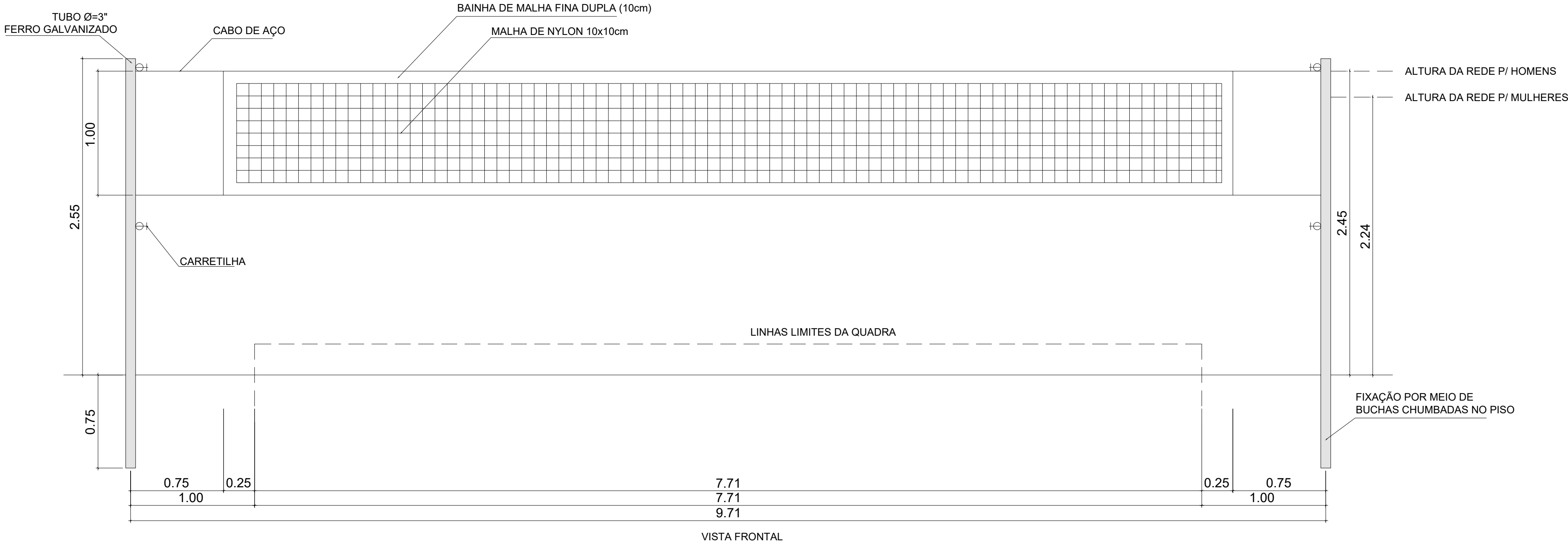
Detalhe 01 - Rede de Vôlei ESC.: 1:25
